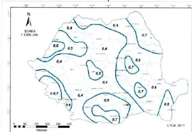
Figura 2.1 Zonarea valorilor de referință ale presiunii dinamice a vântului, q_k în kPa, având AMR = 50 ani NOTA: Pentru altitudin peste 1000m valorile presiunii dinamice a vântului se corectează cu relația (A.1) din Anexa A
