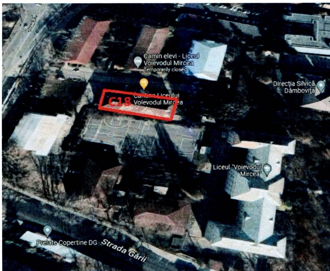
Poziția și datele de identificare ale clădirii analizate pe Google Maps
